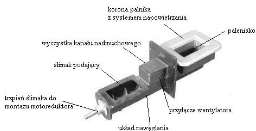
Rys. Budowa układu nawęglania w modelach 50kW i 75kW oraz ECOWARMER Mini 16
