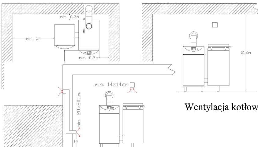
Rys. Usytuowanie kotła
