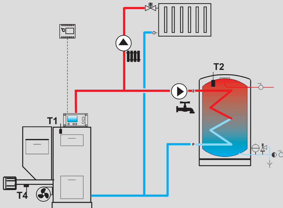
Schemat hydrauliczny ecoMAX 250 RZ
