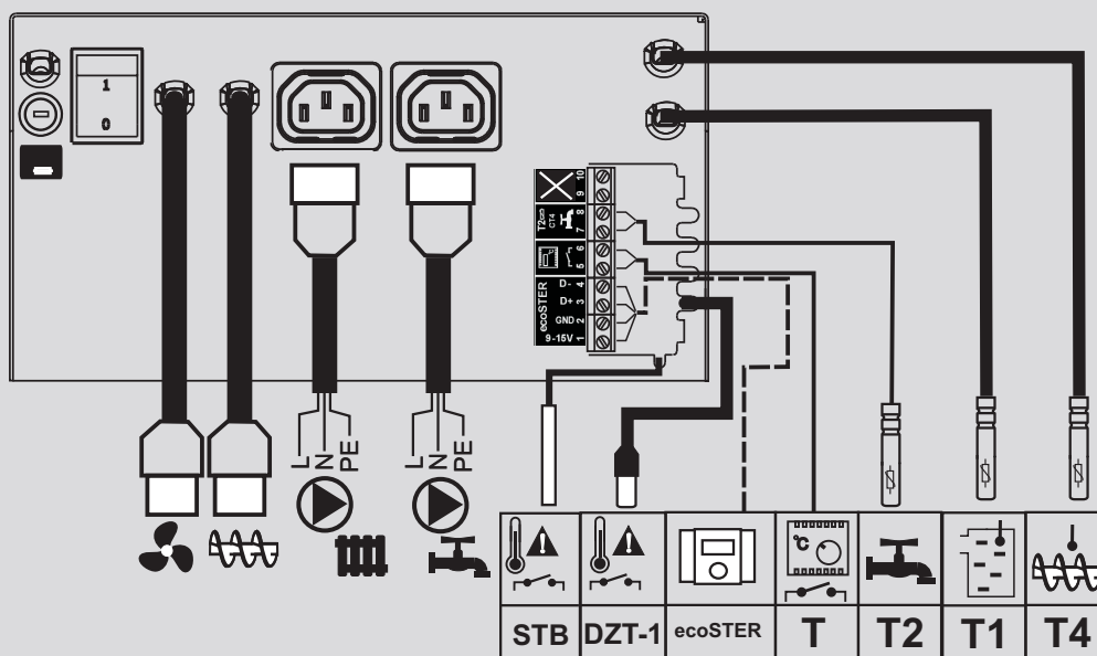
Schemat elektryczny ecoMAX 250 RZ
