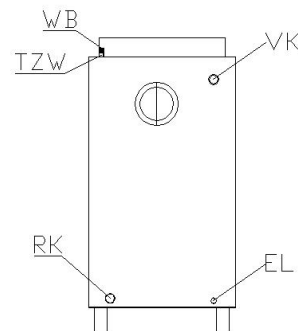
Rys. Rozmieszczenie przyłączy hydraulicznych
