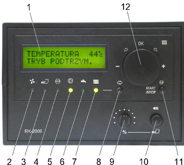
Rysunek 1. Płyta czołowa regulatora RK-2006L2B
